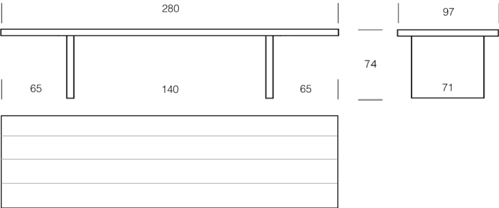
Tischmass table size 280 x 97
